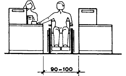
Kasalar arası geçit
