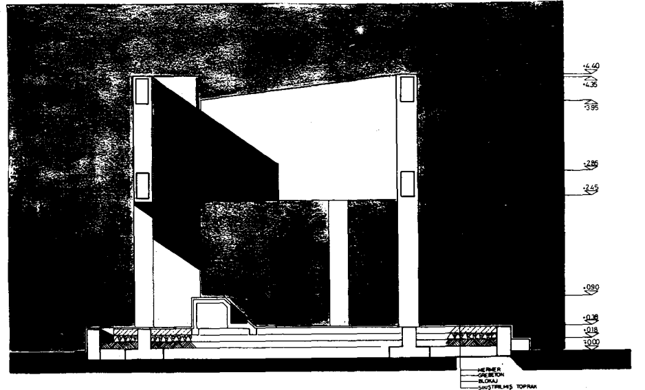
NACI TALAT ANIT MEZARI A-A KESİTİ
