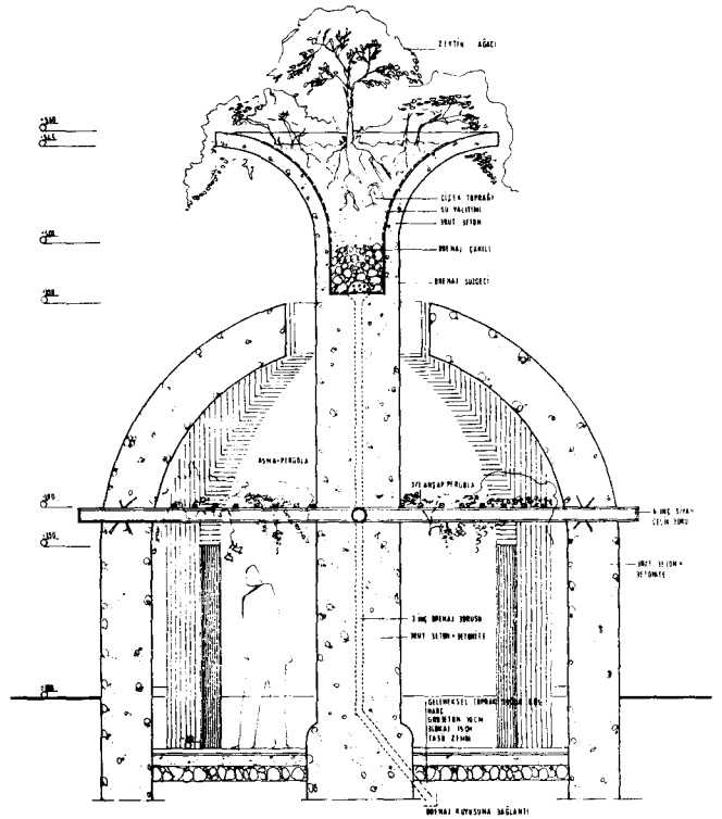
II-II KESİTİ ÖLÇEK : 1/20
